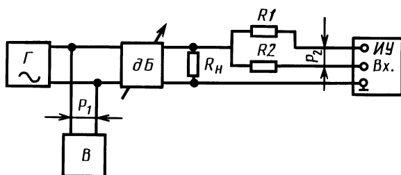
Г — измерительный генератор; дБ — магазин затуханий; В — образцовый измерительный прибор; R1, R2 — резисторы; ИУ — измеритель уровня; Rн — нагрузка магазина затуханий
