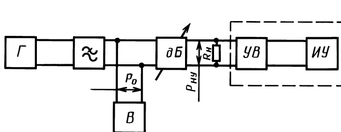
Г — измерительный генератор; ⌘ — фильтр нижних частот; В — образцовый измерительный прибор; дБ — магазин затуханий; УВ — выносное устройство; ИУ — измеритель уровня; Rн — нагрузка магазина затуханий
