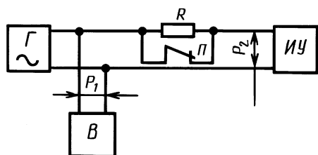
Г — измерительный генератор; R — резистор; П — переключатель; В — образцовый измерительный прибор; ИУ — измеритель уровня
