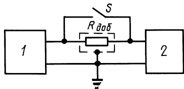
Схема определения входного сопротивления
