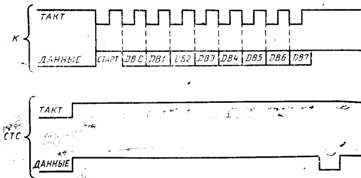
К — клавиатура; СТС — сопрягаемое техническое средство Черт. 1
