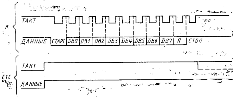
К—клавиатура; СТС—сопрягаемое техническое средство. Черт. 2
