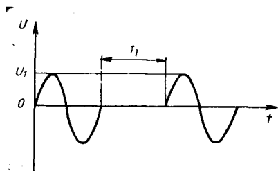
Форма сигнала прерывания переменного напряжения
