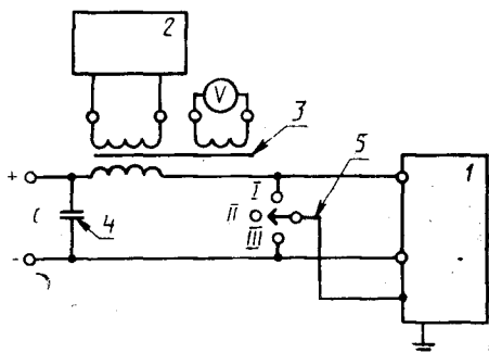
1 — испытуемое изделие; 2 — генератор; 3 — соединительный трансформатор; 4 — конденсатор, C=47 мкФ; 5 — переключатель (I и III — несимметричная помеха, II — симметричная помеха)
