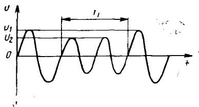
Форма сигнала провала переменного напряжения
