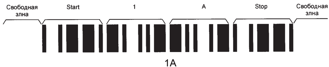
Рисунок 1. Символ Code 39
