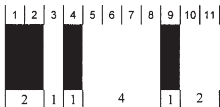
Рисунок 2 — Знак Start A для Code 128
