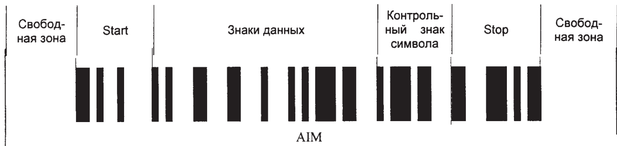
Рисунок 1 — Символ Code 128
