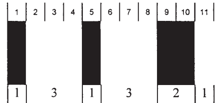
Рисунок 3 — Знак символа для значения 35
