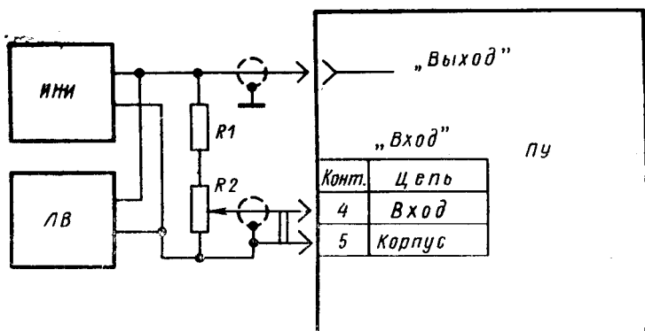
Схема для проверки нелинейных искажений
