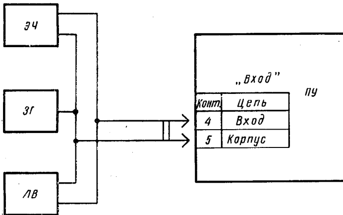
Схема для проверки погрешности измерения перемещения
