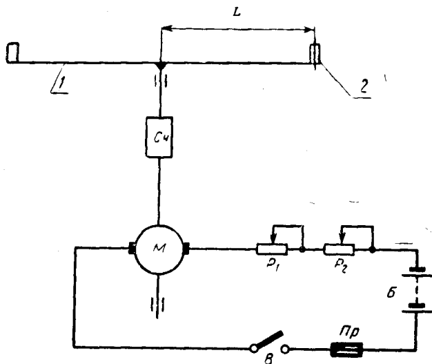
1—крестовина; 2—стойка для крепления проверяемых анемометров; Сч—счетчик числа оборотов крестовины; М—двигатель; P_1 , P_2 —реостаты; Б—аккумуляторная батарея; В—выключатель; Пр—предохранитель.
