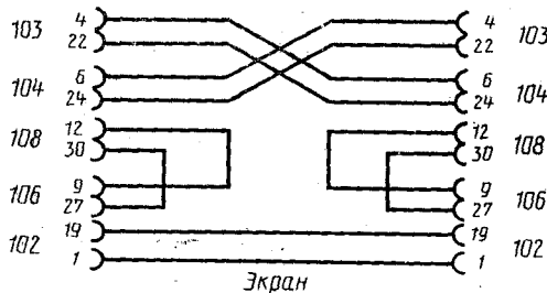
Соединение контактов
