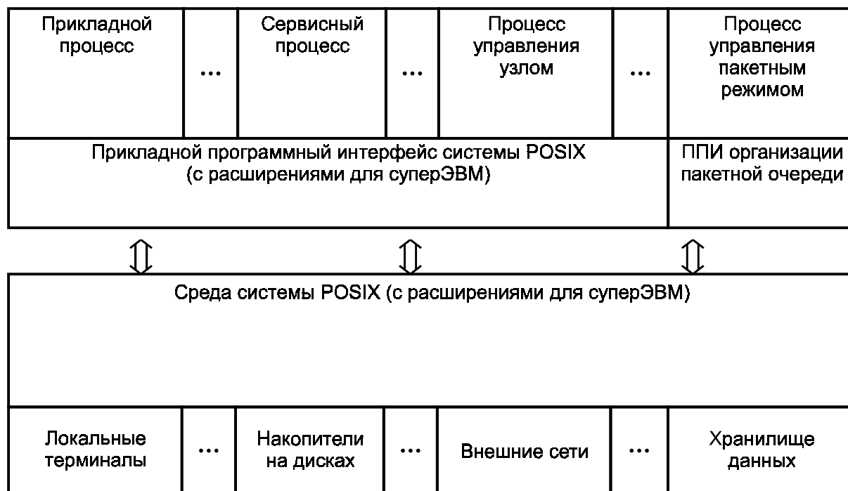
Рисунок 1 — Модель среды суперЭВМ на основе POSIX
