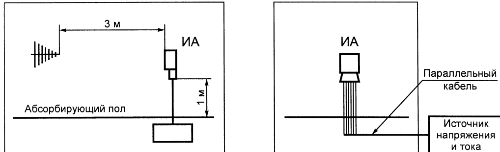
Рисунок Е.1 — Установка для проведения испытаний на устойчивость к электромагнитным радиочастотным полям
