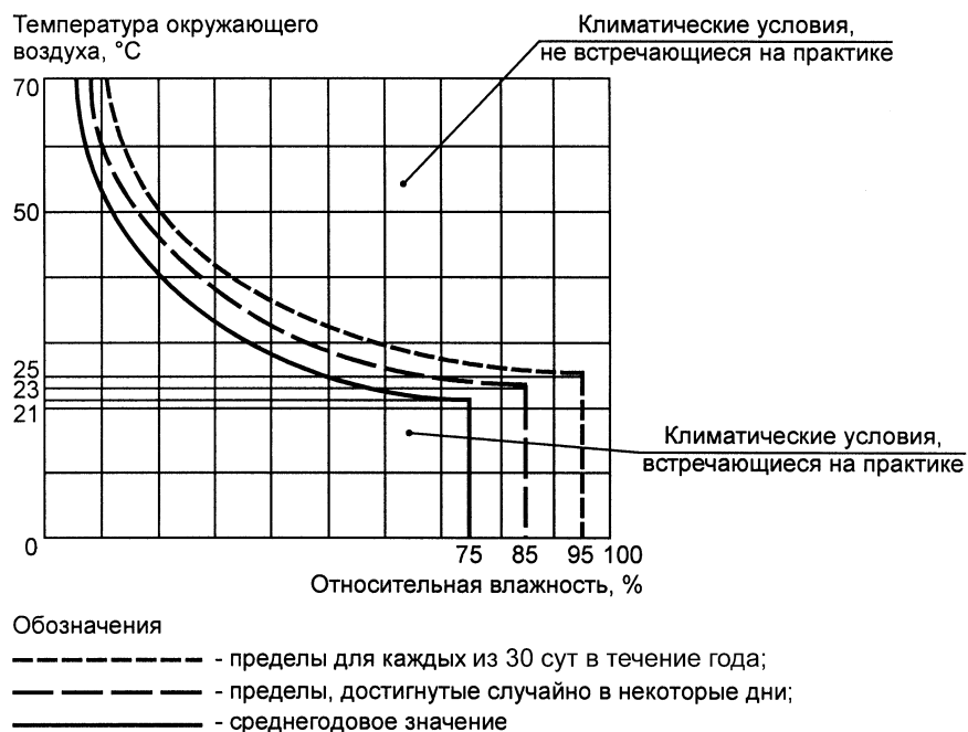
Рисунок А.1 — Соотношение между температурой окружающего воздуха и относительной влажностью
