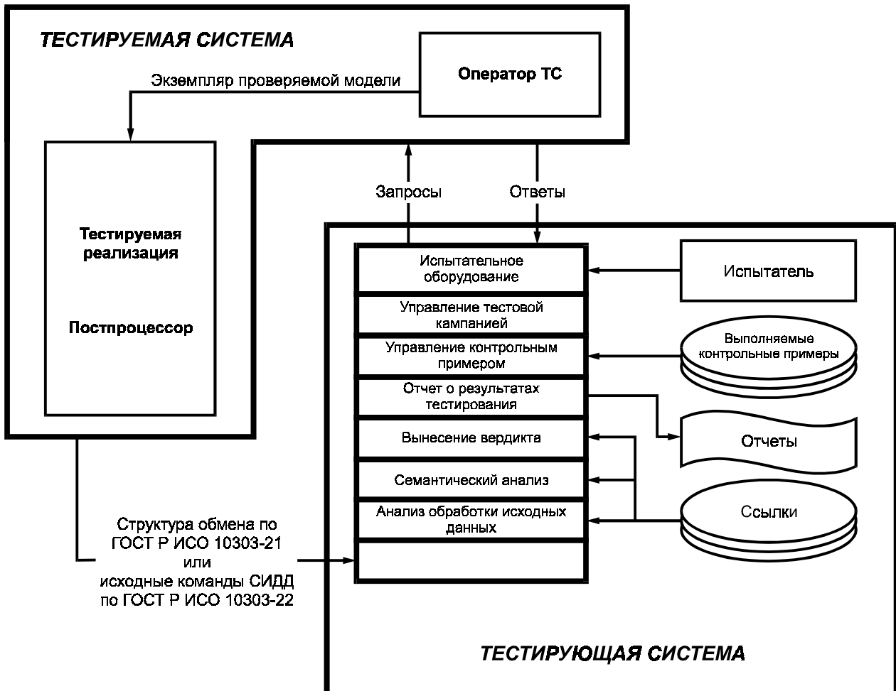
Рисунок 2 — Компоненты тестирования постпроцессора
