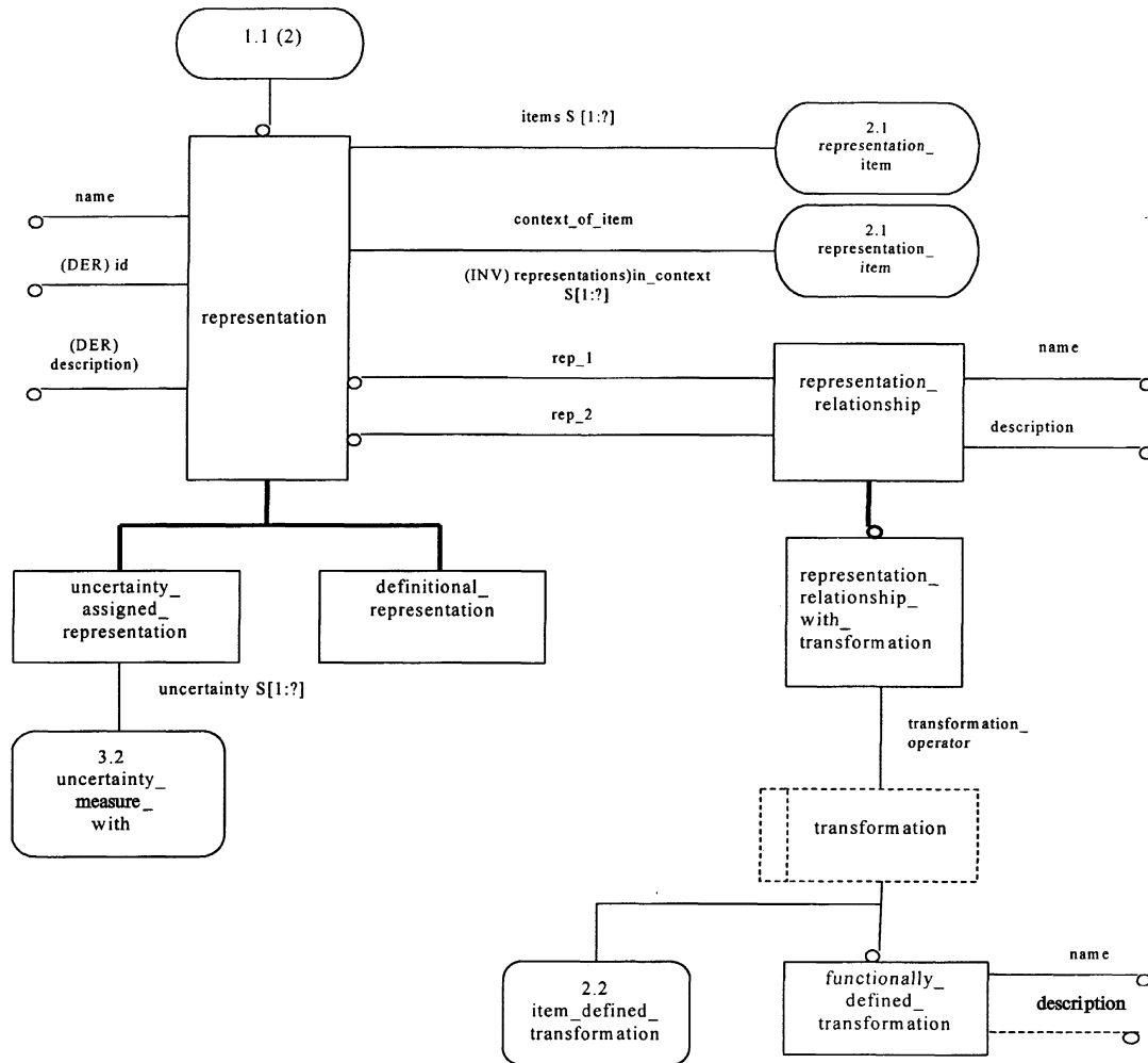
Рисунок D.1 — EXPRESS-G диаграмма representation_schema 1 из 3
