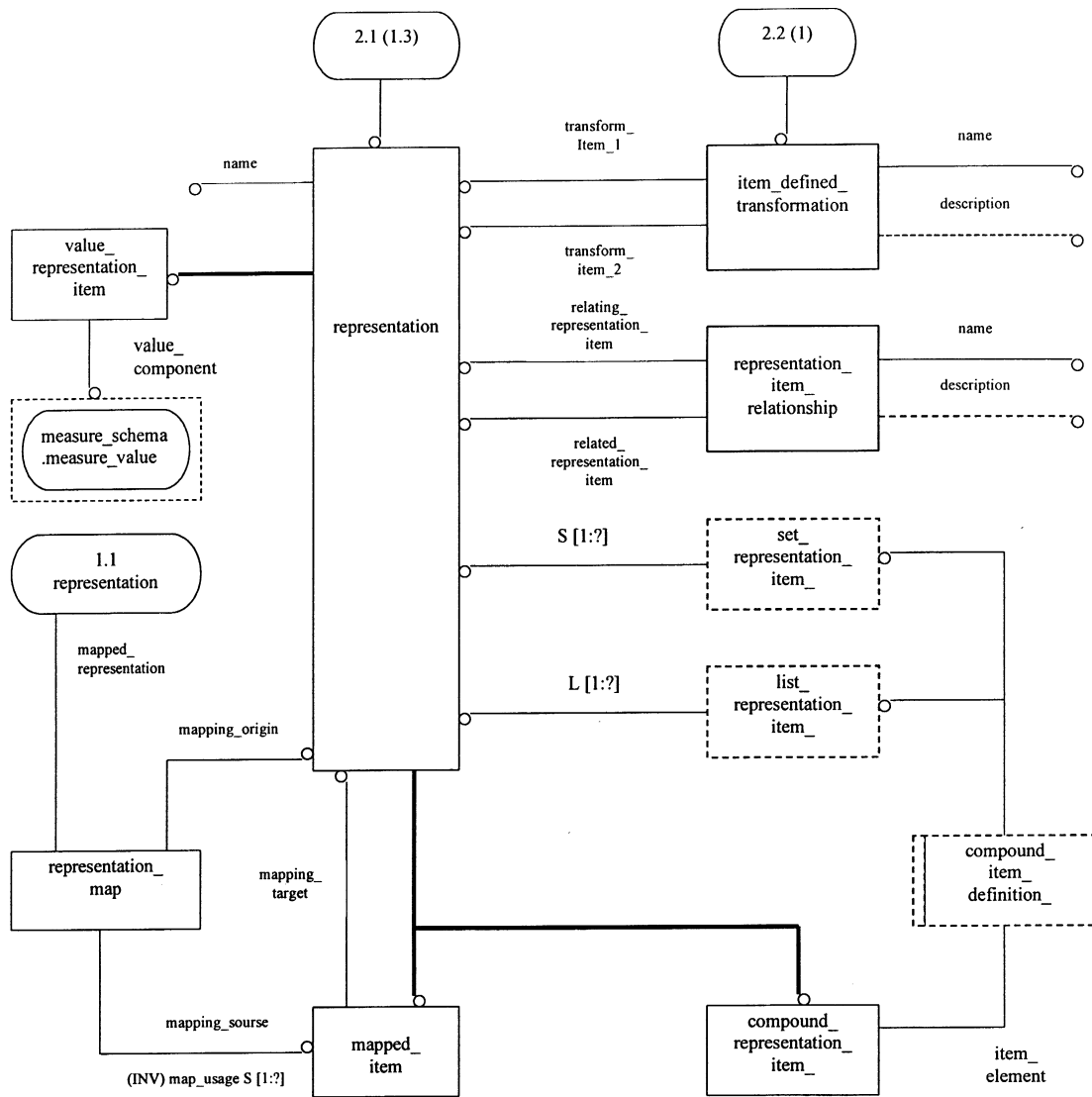
Рисунок D.2 — EXPRESS-G диаграмма representation_schema 2 из 3
