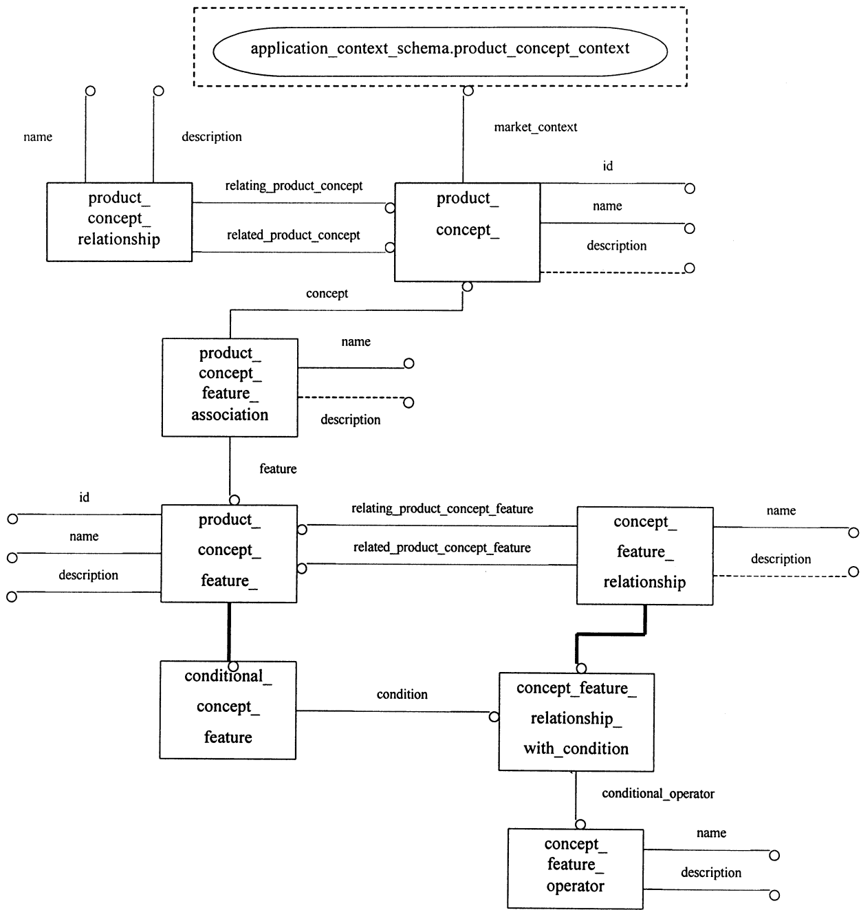
Рисунок D.2 — product_concept_schema
