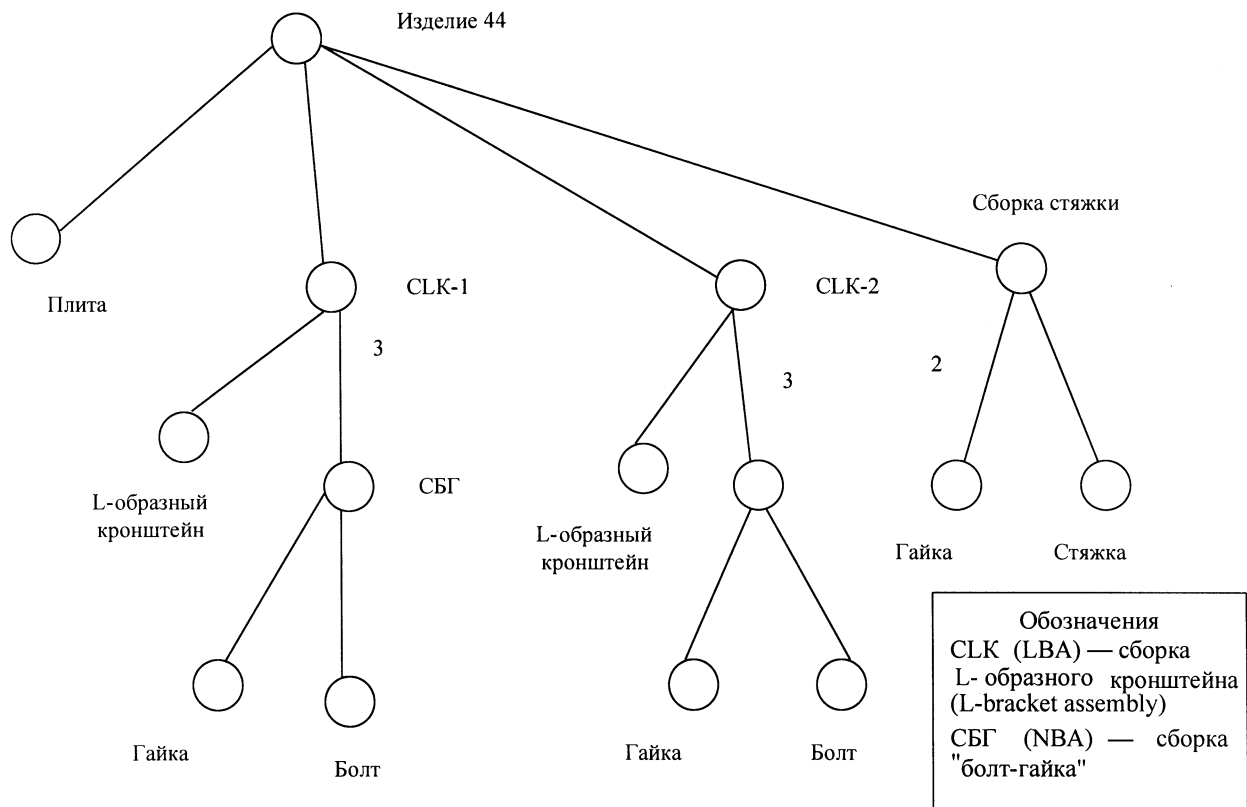
Рисунок Е.2 — Схематическое представление структуры «изделия 44»
