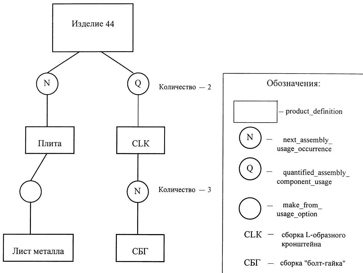
Рисунок Е.5 — Пример структуры данных СП с использованием объектов настоящего стандарта
