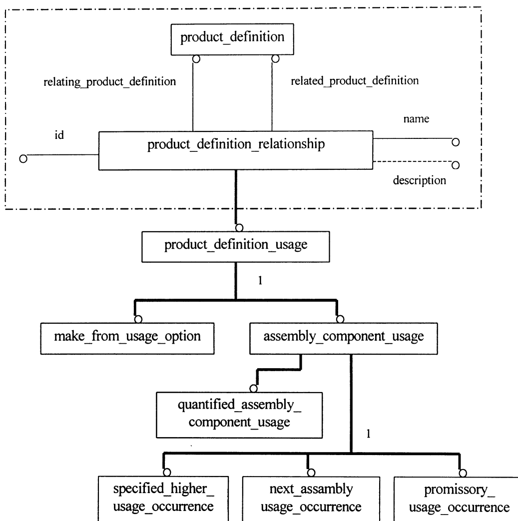
Рисунок 2 — Взаимосвязь объектов структуры изделия по ИСО 10303-41
