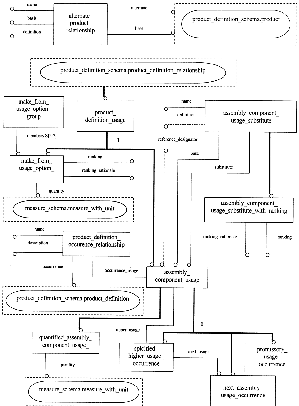
Рисунок D.1 — product_structure_schema
