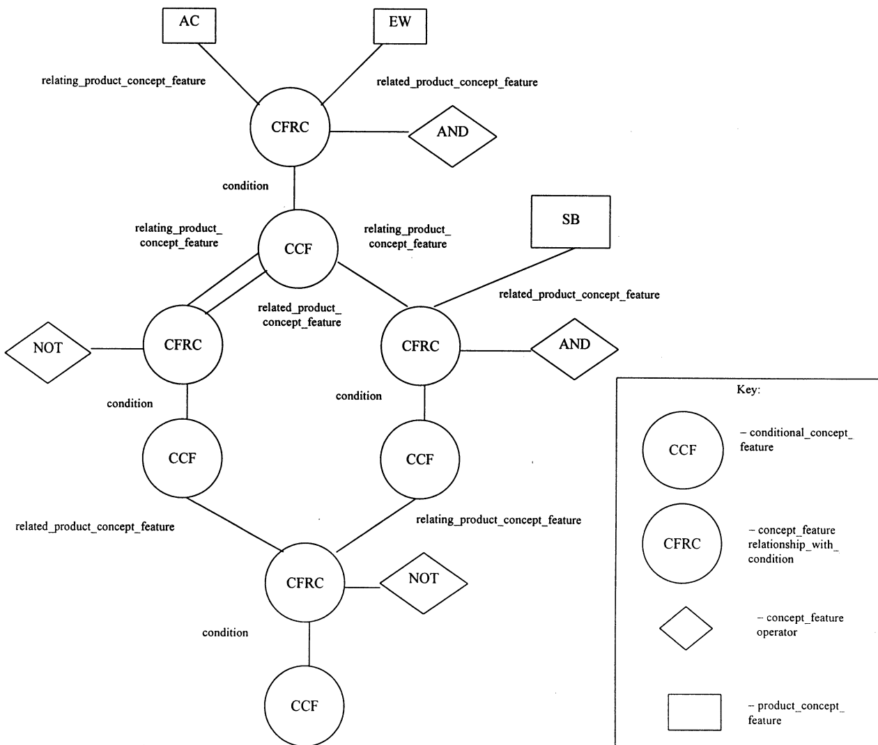
Рисунок E.13 — Двоичные операторы для conditional_concept_feature
