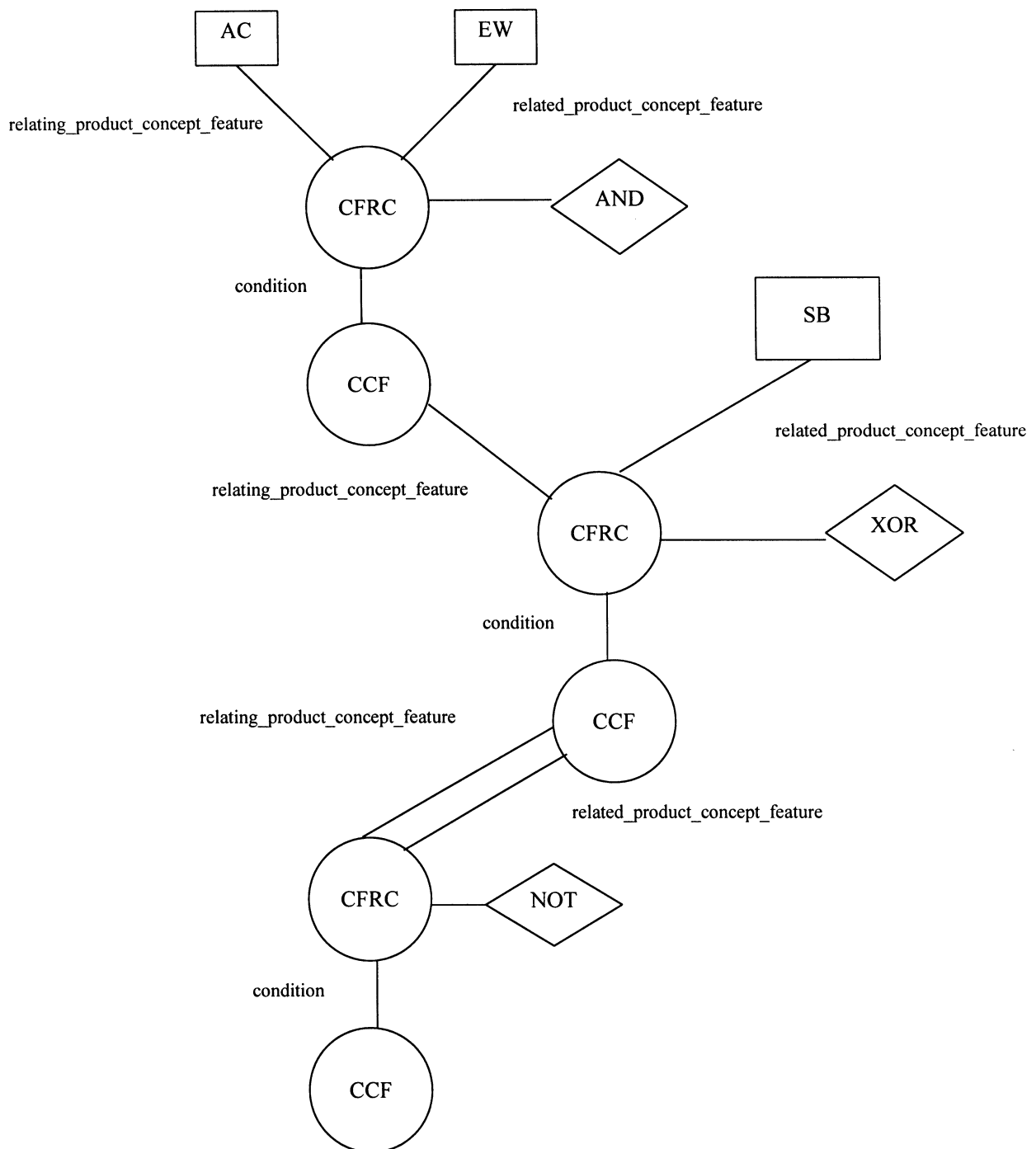
Рисунок Е.12 — Альтернативные двоичные операторы для conditional_concept_feature
