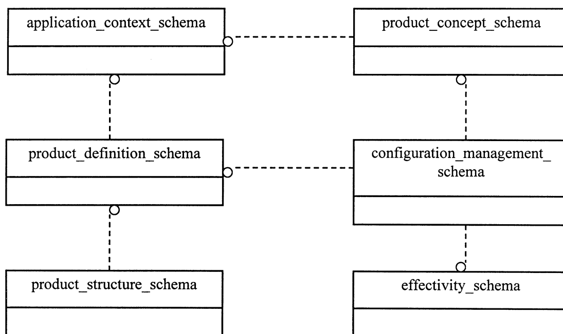
Рисунок 1 — Отношения схем интегрированных ресурсов
