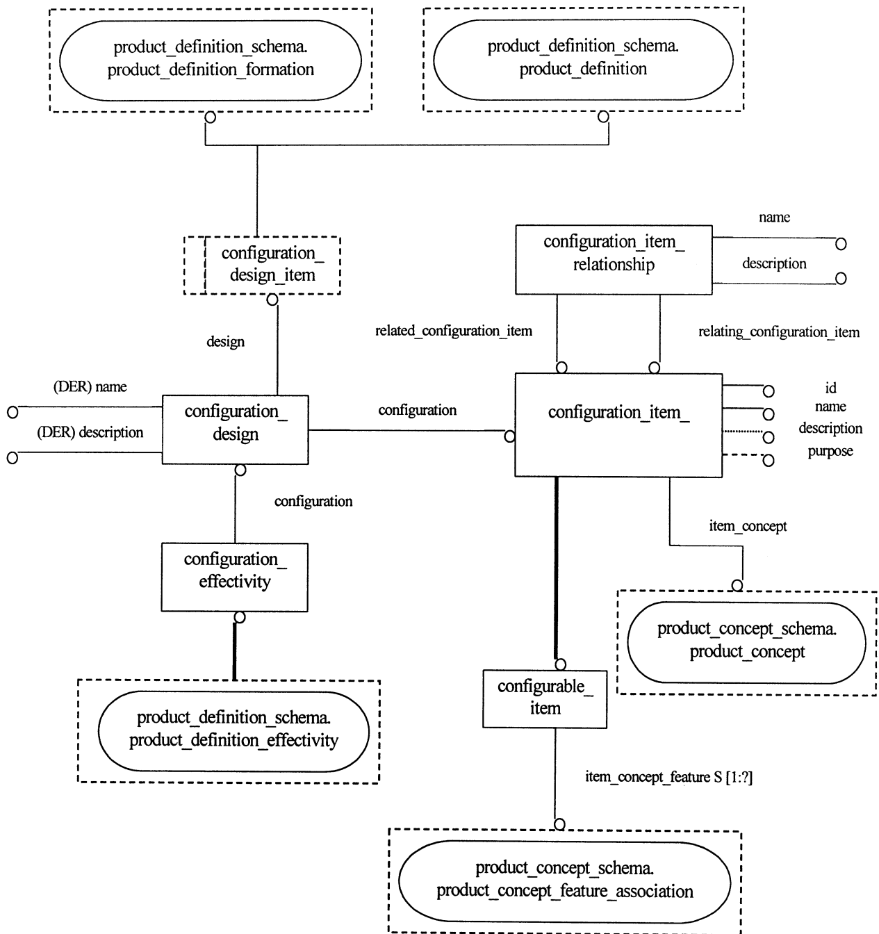
Рисунок D.3 — configuration_management_schema
