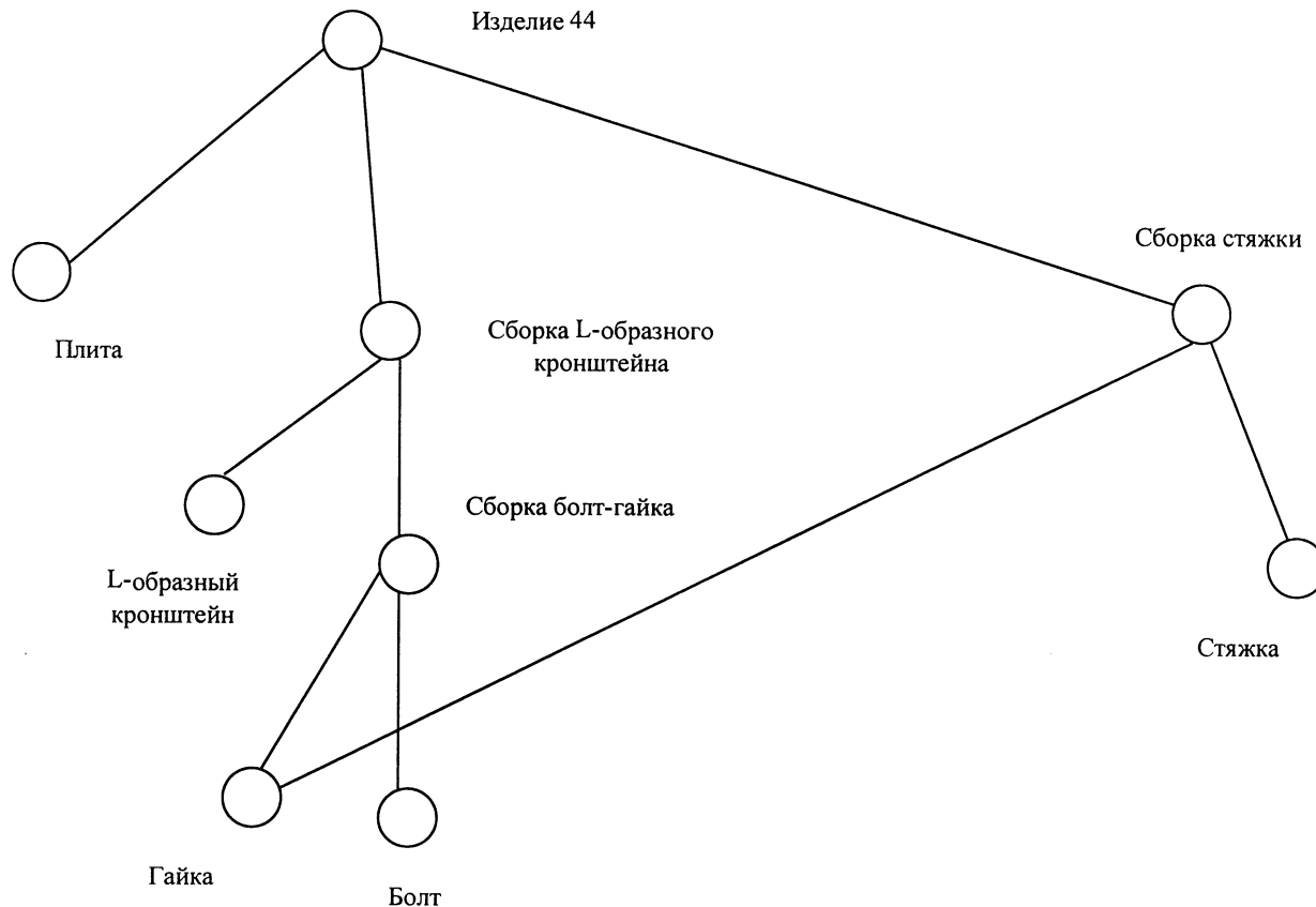
Рисунок Е.3 — Структура данных СП для изделия 44
