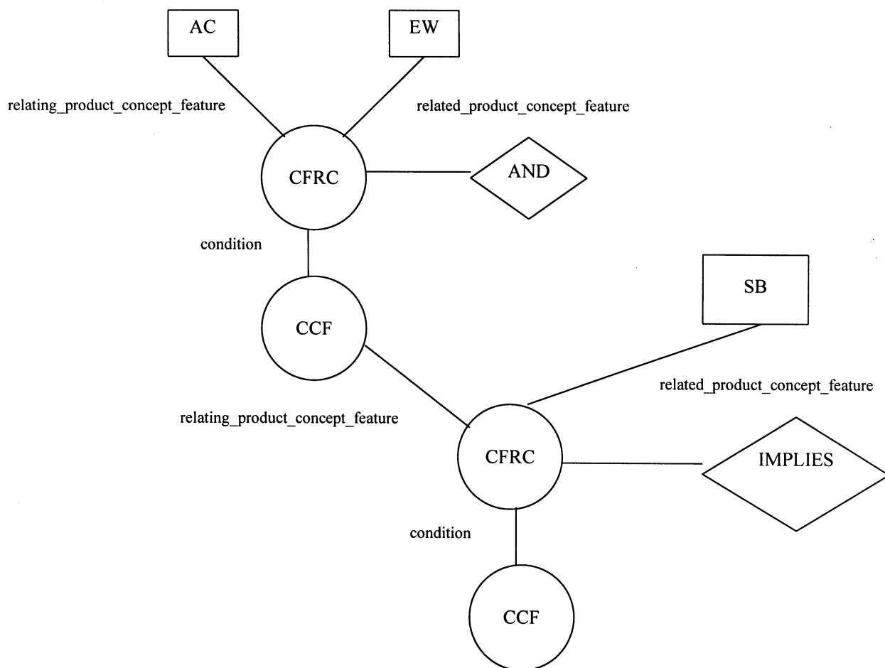
Рисунок E.14 — Определенные операторы для conditional_concept_feature
