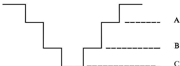
Рисунок Е.1 — Операция сверления
