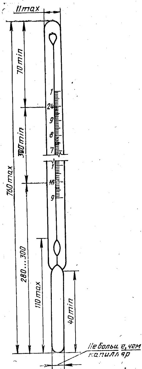
Рисунок 1 — Термометр палочный калориметрический
