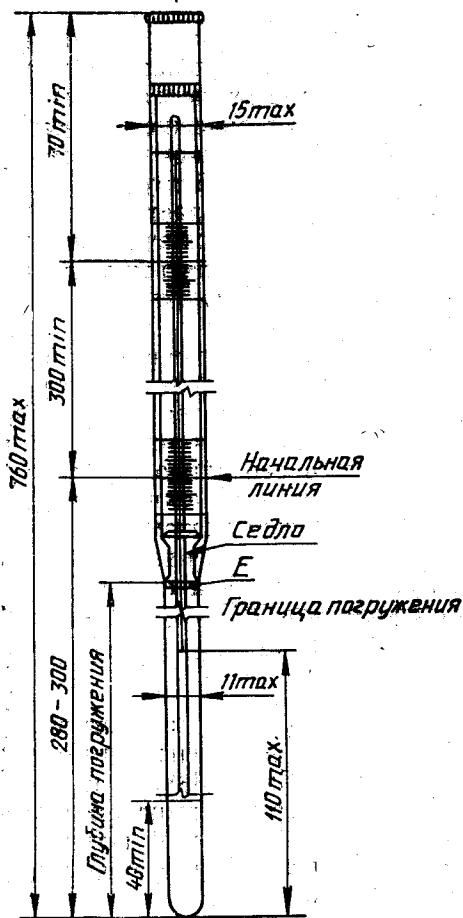
Рисунок 1 — Термометр с вложенной шкалой калориметрический
