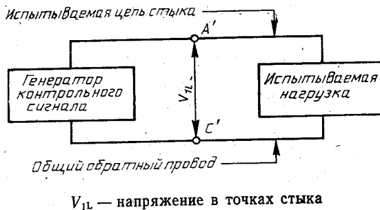
Рисунок 4 — Испытательная схема нагрузки V.10
