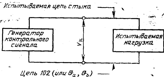
Рисунок 2 — Испытательная схема нагрузки V.28
