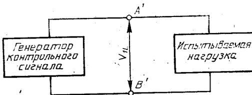
Рисунок 6 — Испытательная схема нагрузки V.11
