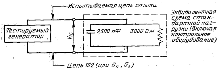
Рисунок 1 — Испытательная схема генератора V.28
