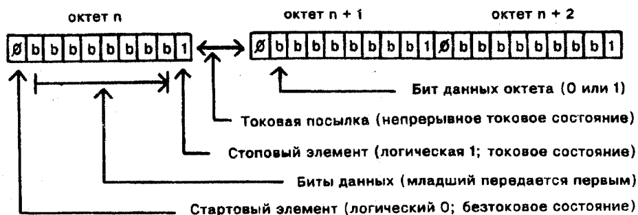
Рисунок 2 — Типичная передача октета при стартстопной передаче
