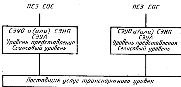
Рисунок 1 — Модель обеспечивающих уровней
