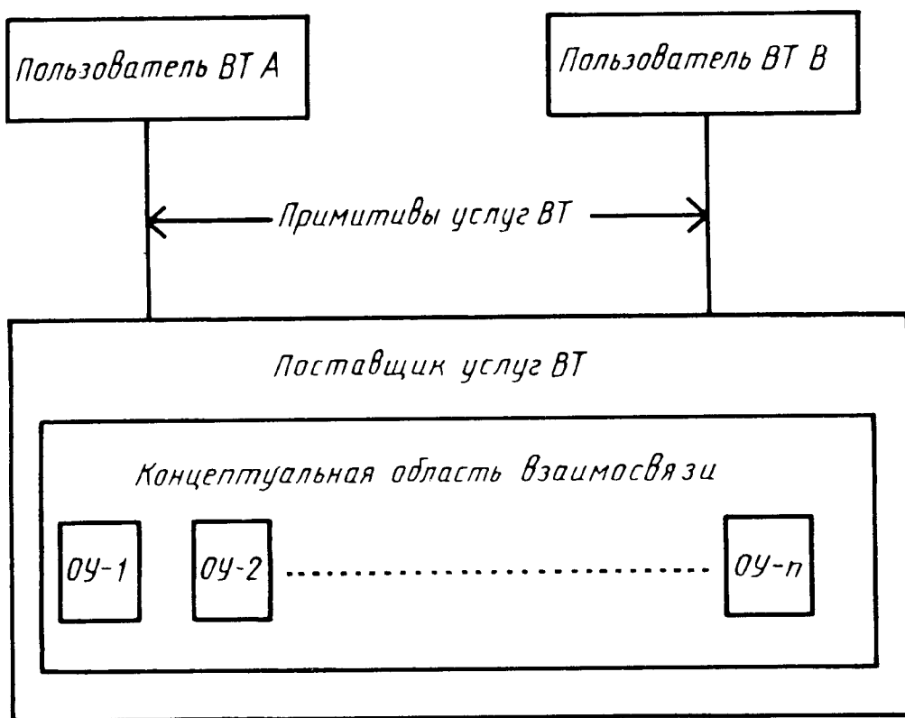
Рисунок 1 — Объекты управления в модели услуг ВТ
