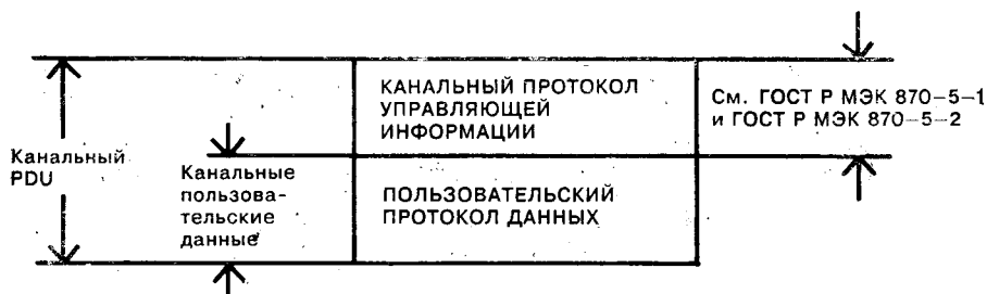
Рисунок 3 — Структура кадра для модели 2
